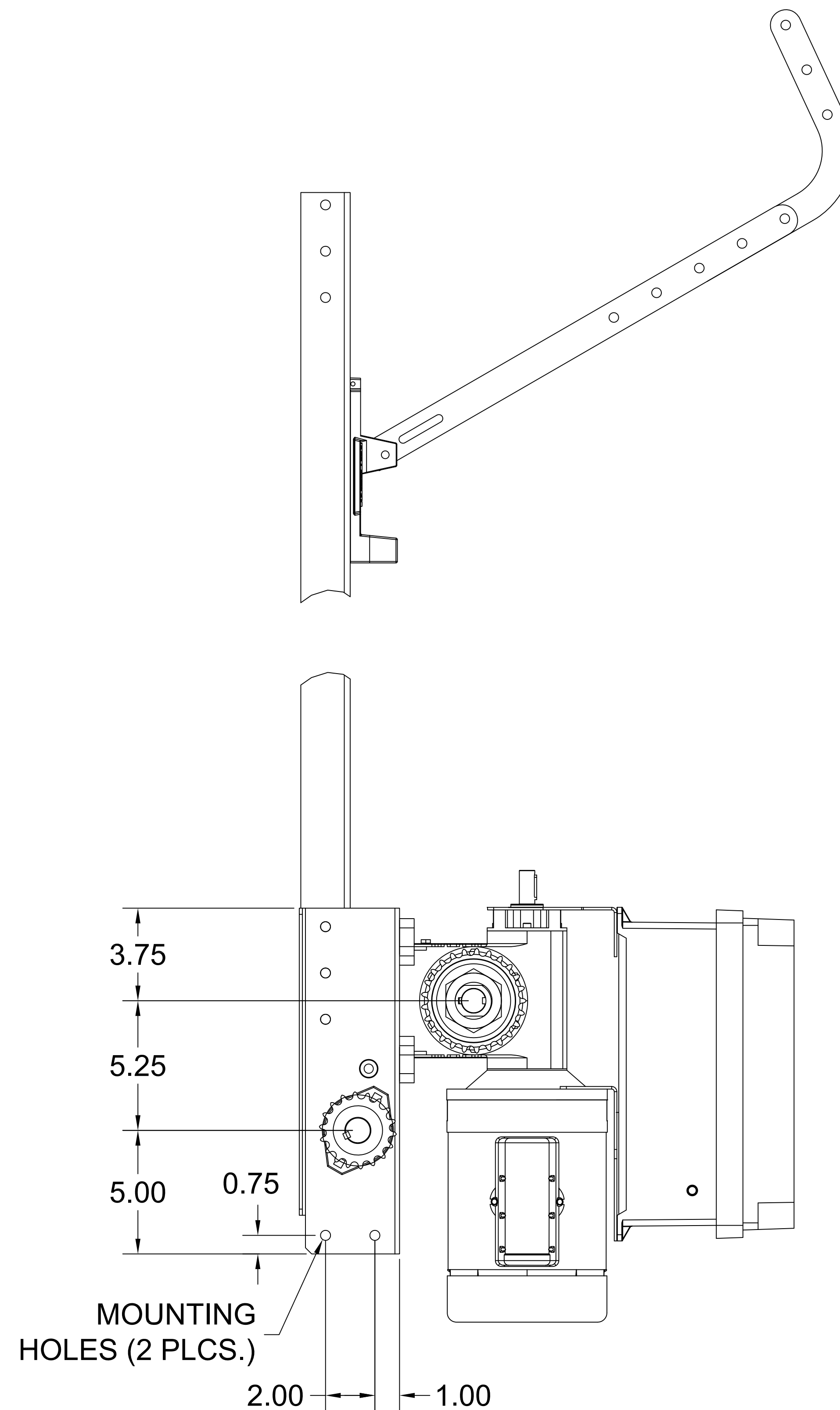
LEFT
