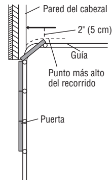
Puerta seccional con guía curva
