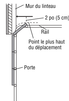
Porte sectionnelle avec rail incurvé
